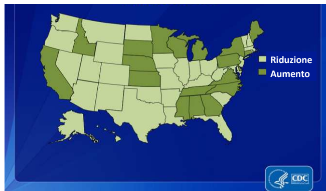
Trend delle notifiche di Pertosse negli USA dal 2013 al 2014 (tratto da www.cdc.gov )
